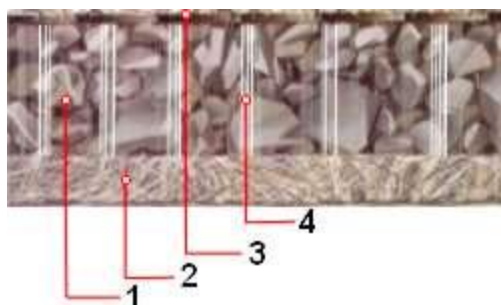
Рисунок 2. Строение геотекстиля марки «KAZGEOBEL-1»
